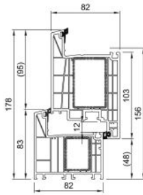
PRZEKRÓJ RAMA-SKRZYDŁO
