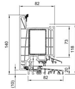
PRZEKRÓJ SKRZYDŁO-PRÓG
